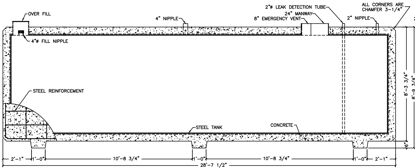
SECTION A-A
