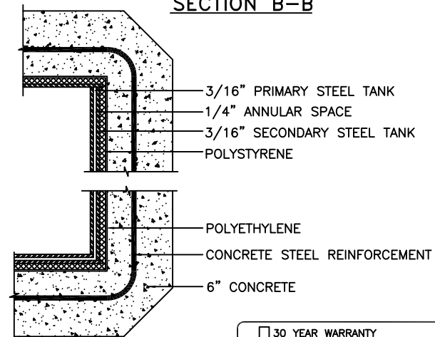
CORNER DETAILS N.T.S.
