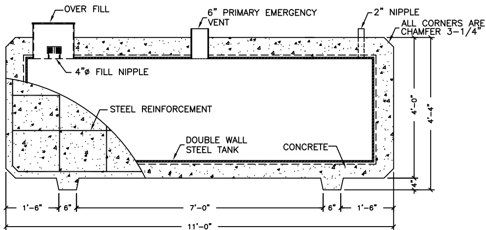
SECTION A-A
