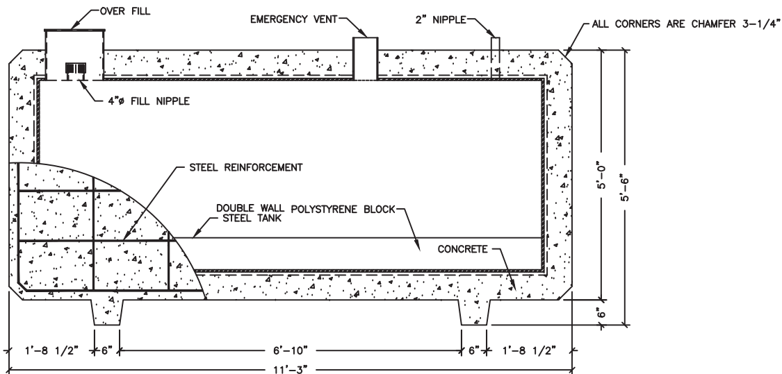
SECTION A-A
