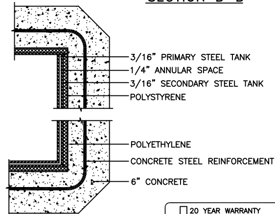
CORNER DETAILS N.T.S.
