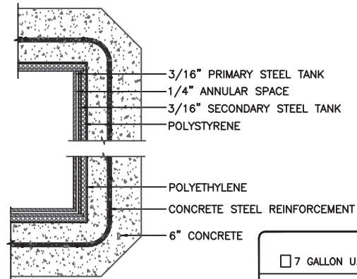
CORNER DETAILS N.T.S.
