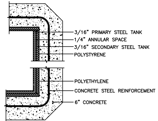
CORNER DETAILS N.T.S.
