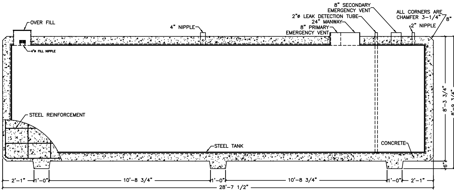
SECTION A-A
