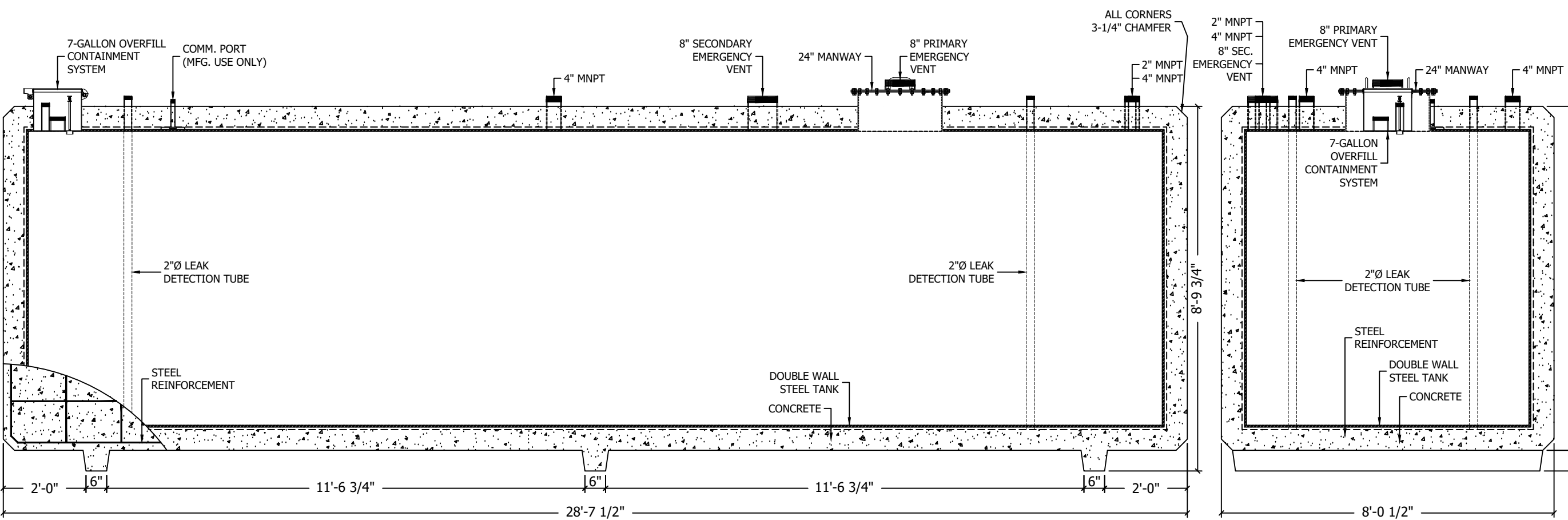
SECTION A-A
